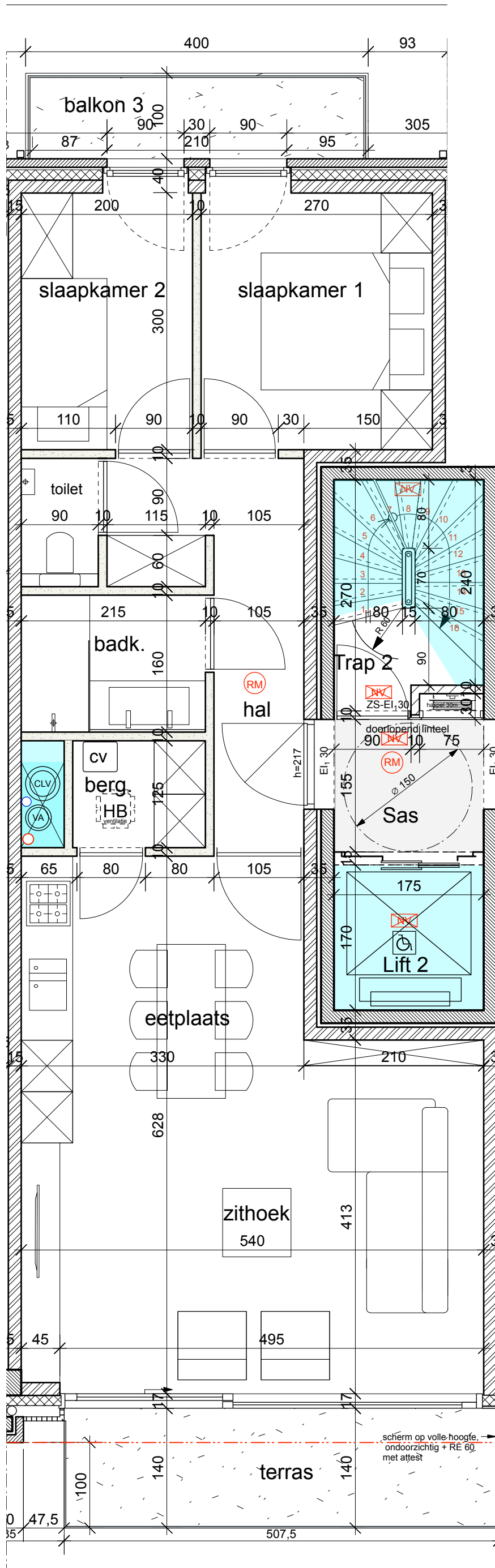
appartement 62.03.01: 68 m 2 + 11 m 2 terrassen
