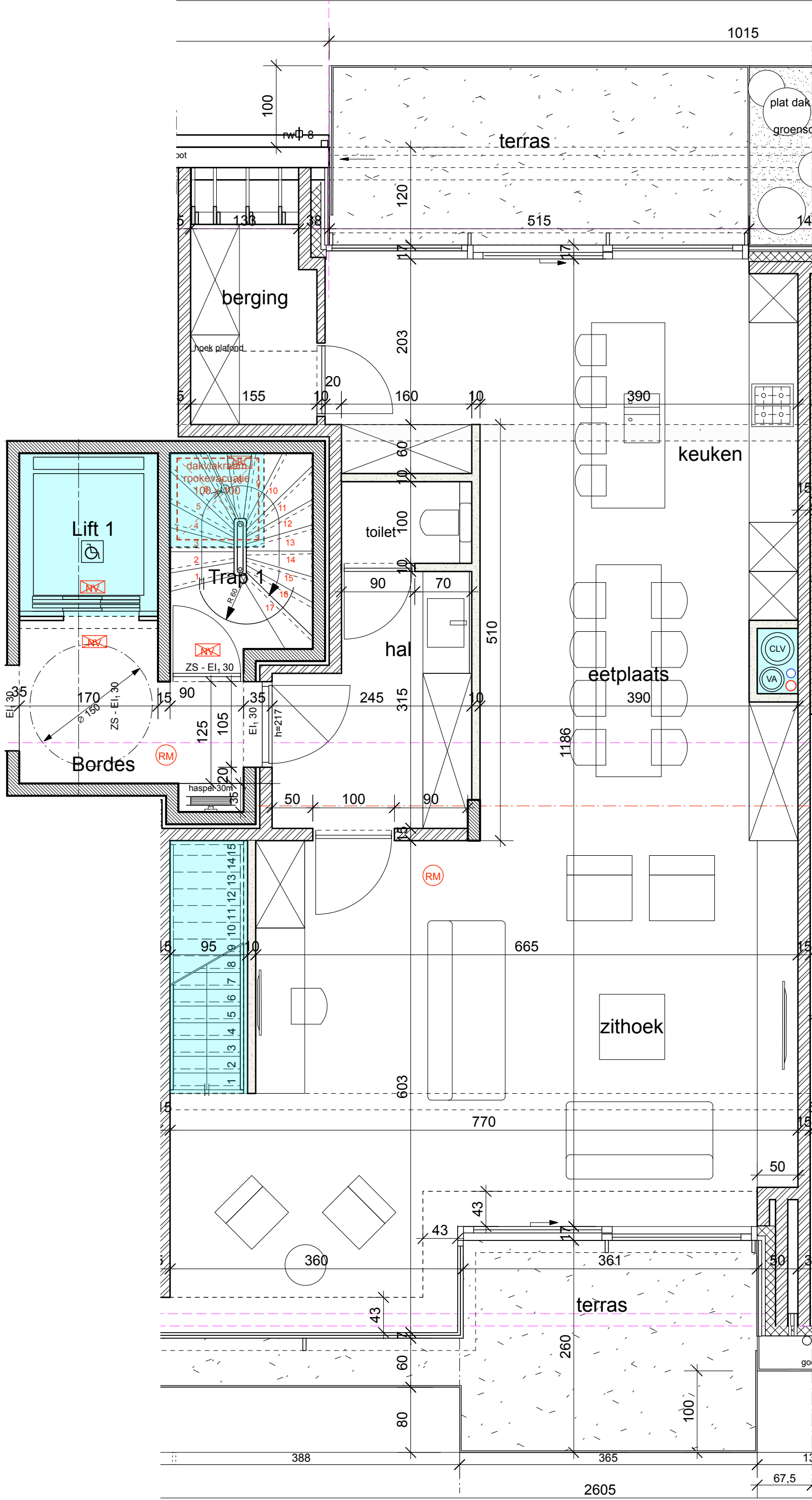
appartement 60.05.01: 148 m 2 + 23 m 2 terrassen
